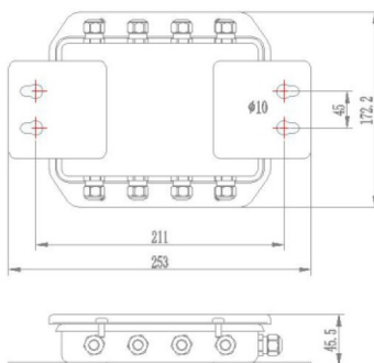
六进一出、八进一出尺寸图
