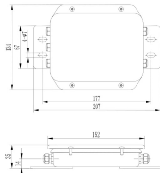
四进一出尺寸图
